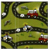
98. 소아 온더로드
